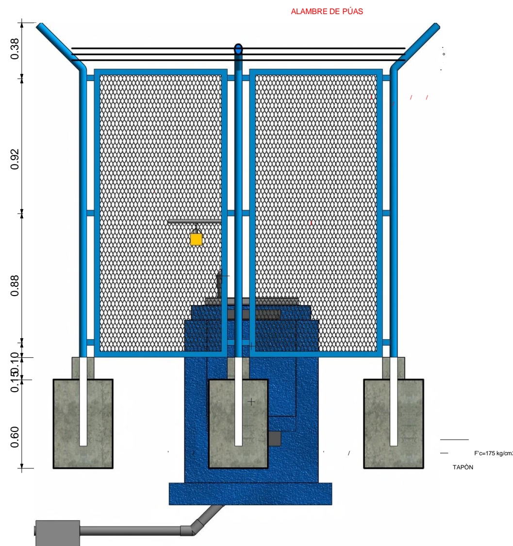
CÁMARA ROMPE PRESIÓN 6 - CORTE B'-B' ESC. 1:15
