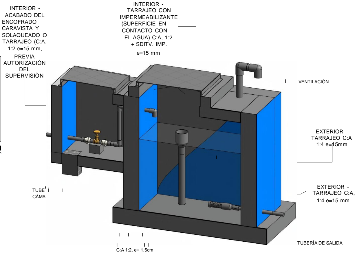
CÁMARA ROMPE PRESIÓN 6: CORTE EN SECCIÓN 3D ESC. 1:10
