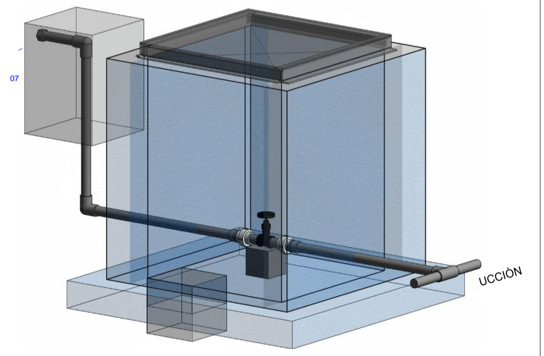
IS VÁLVULA DE AIRE: VISTA 3D ESC. 1:10
