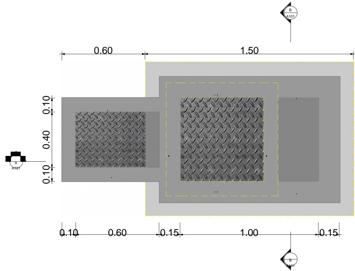
CÁMARA ROMPE PRESIÓN 6: VISTA EM PLANTA ESC. 1:10
