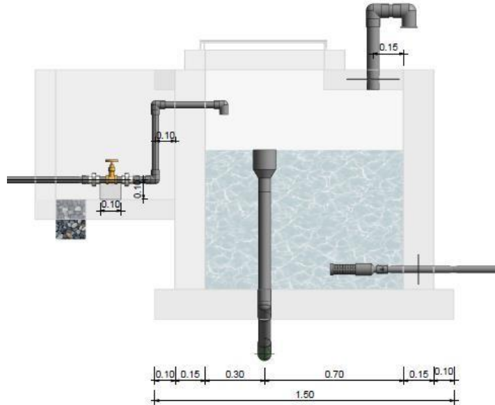
Figura 10 Cámara rompe presión tipo 6 Fuente: Dominguez Z.
