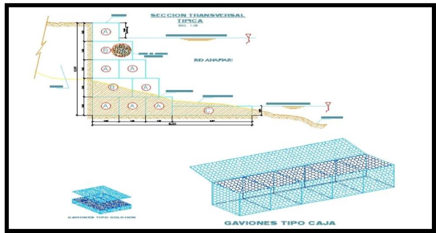
Figura 12: Diseño constructivo y estructural de varios detalles de gaviones
