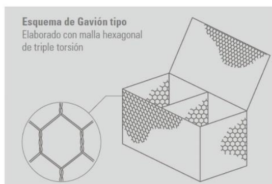
Figura 3. Esquema de Gavión tipo caja. Fuente:(A Bianchini, 2017).
