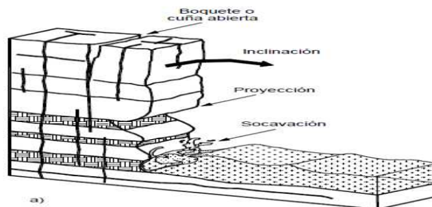
Figura 13: Proceso de socavación.
