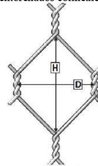
Figura 7. Dimensionamiento malla triple torsión para talud. Fuente: Fichas Técnicas Aceros Metales y Mallas Ltda.
