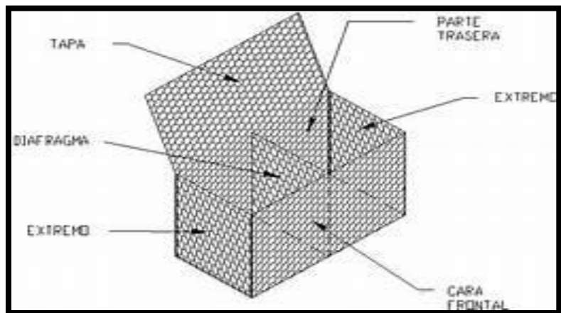
Figura 5: Gavión tipo Caja
