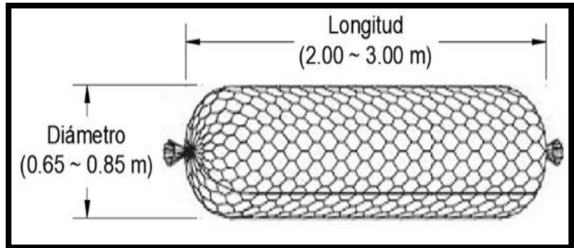
Figura 6: Gavión tipo Saco
