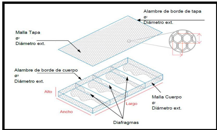
Figura 7: Gavión tipo colchón
