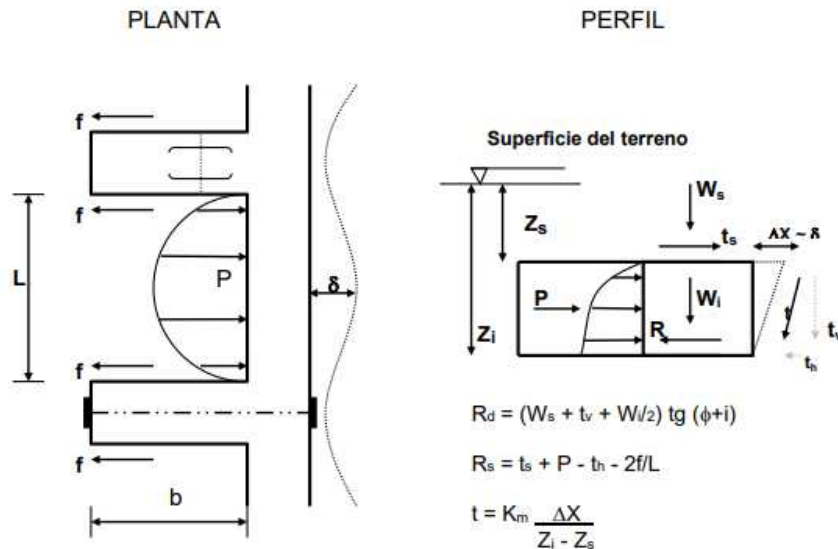
FIGURA N° 8: DIAGRAMA DE CUERPO LIBRE DE UN MURO DE GAVIONES CON CONTRAFUERTE
