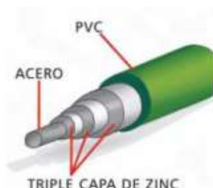
Figura 10. Recubrimiento del alambre de la malla de gaviones 4 .
