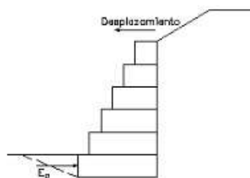
Figura 18. Efecto del empuje pasivo 2 .
