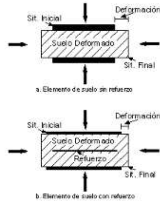
Figura 26. Deformaciones en elementos de suelo con y sin refuerzo 7 .
