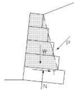
Figura 25. Análisis de la estabilidad interna de muros de gaviones 3 .
