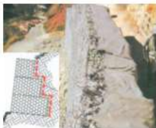
Figura 38. Uso de geotextil en gaviones 10 .
