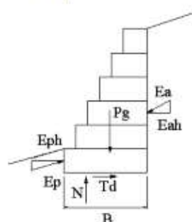
Figura 20. Verificación de estabilidad contra el deslizamiento 3 .
