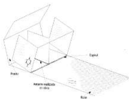
Figura 28. Elemento Terramesh System 8 .
