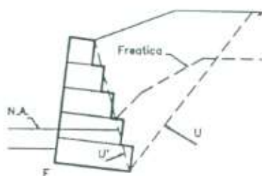
Figura 17. Presiones generadas por la superficie freática 3 .
