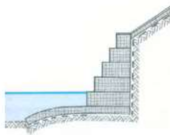
Figura 32. Obras longitudinales macizas 8 .
