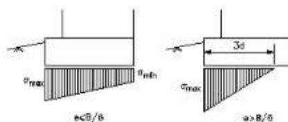
Figura 22. Distribución de presiones en la base del muro 3 .
