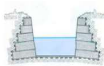
Figura 35. Canalización a base de colchones y gaviones 3 .
