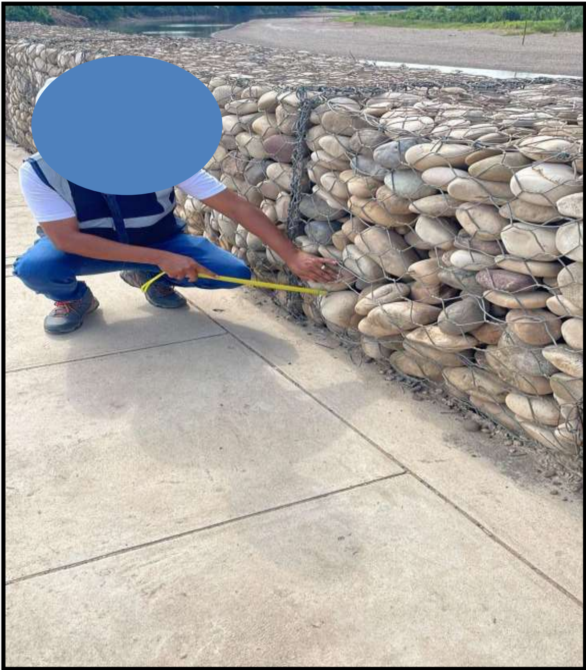
Figura 26: Rotura de malla de gavión
