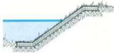
Figura 31. Obras longitudinales leves 8 .
