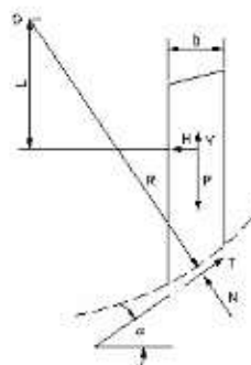
Figura 24. Geometría y fuerzas que actúan en las dovelas 3 .
