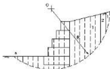
Figura 23. Método de las dovelas 3 .
