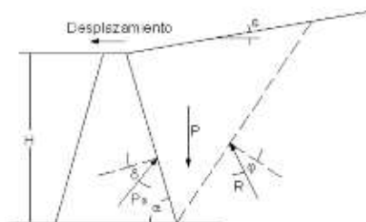
Figura 14. Fuerzas actuantes sobre la cuña de suelo 3 .
