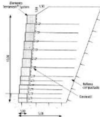
Figura 27. Sección transversal típica de una estructura de Terramesh 8 .
