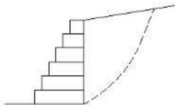
Figura 13. Superficie de rotura 3 .
