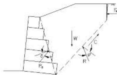
Figura 15. Fuerzas actuantes sobre la cuña de suelo cohesivo 3 .
