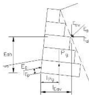
Figura 21. Verificación de la estabilidad contra el vuelco 3
