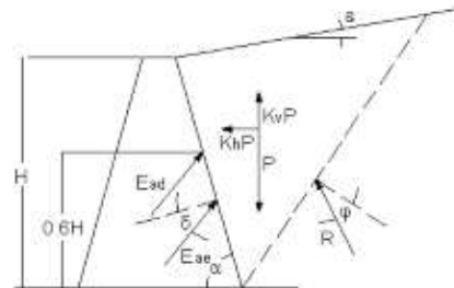
Figura 16. Fuerzas debidas al sismo 3 .
