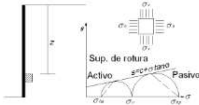
Figura 12. Determinación de la presión horizontal 2 .
