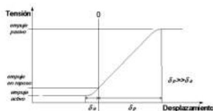
Figura 11. Empuje de suelo sobre un elemento móvil 7 .
