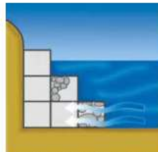
Figura 9. Permeabilidad de los muros de gaviones 4 .
