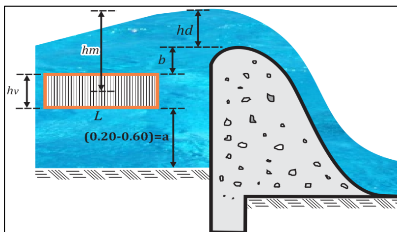
Figura 24: diseño de la ventana de captación
