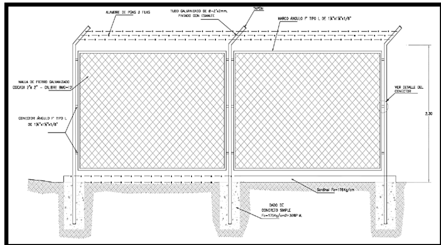
Figura 18: Cerco para reservorio
