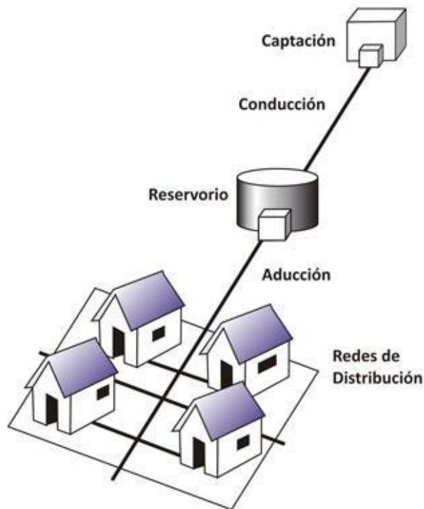
Figura 1: Sistema por gravedad sin tratamiento Fuente: OPS 2013
