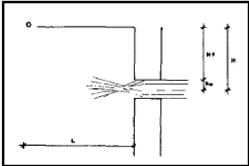
Figura 12: Pérdida de carga y Carga disponible Fuente: Agüero R., (1997)
