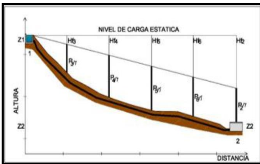
Figura 7: Calculo de la línea de gradiente hidráulica (LGH)
