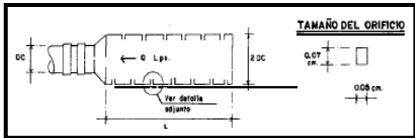
Figura 15: Canastilla de salida
