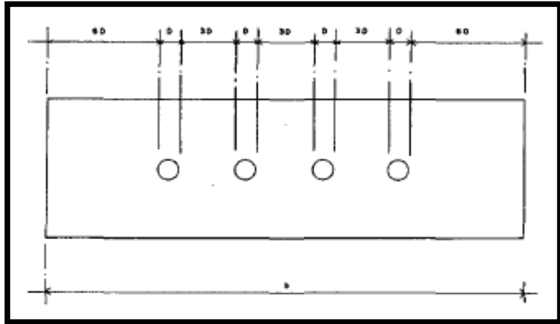
Figura 13: Distribución de los orificios (pantalla frontal)
