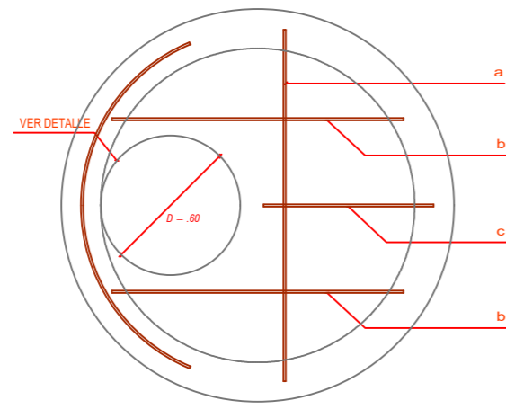
ARMADURA INFERIOR LOSA DE TECHO fc = 210 kg/cm 2
