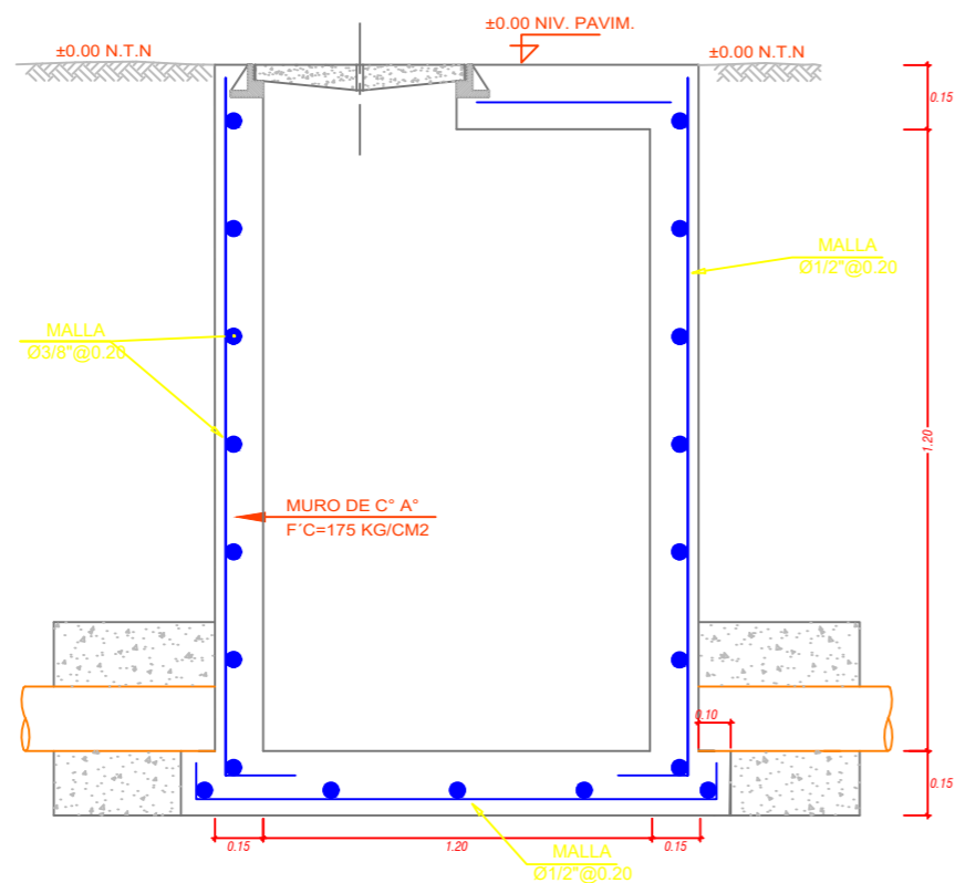
DETALLE DE CAMARA DE INSPECCION ESC: 1/20
