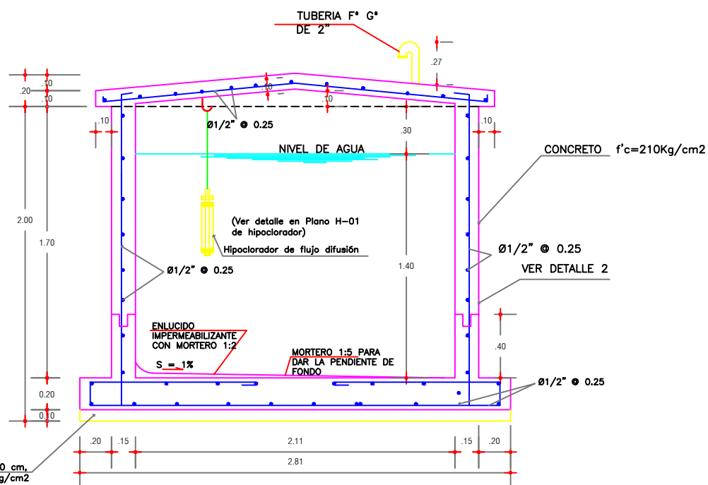
CORTE A - A ESC: 1/10
