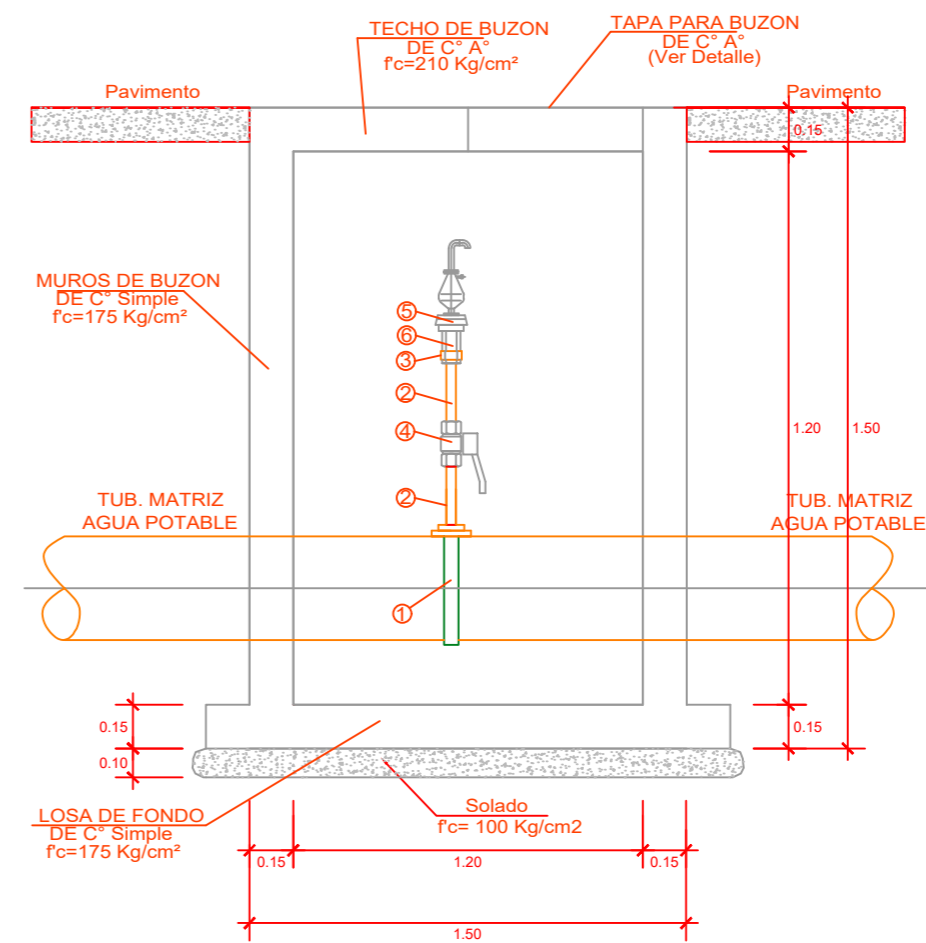
CORTE C-C
