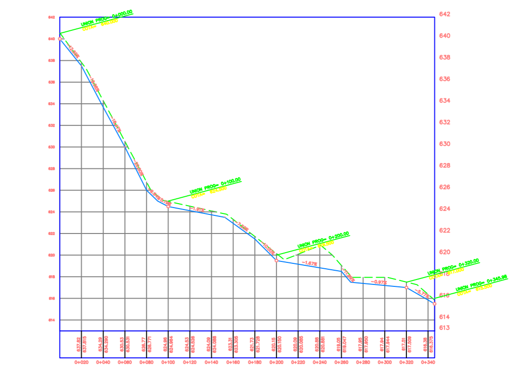
PERFIL DE LA LINEA DE RED DISTRIBUCION SECUNDARIA 4
