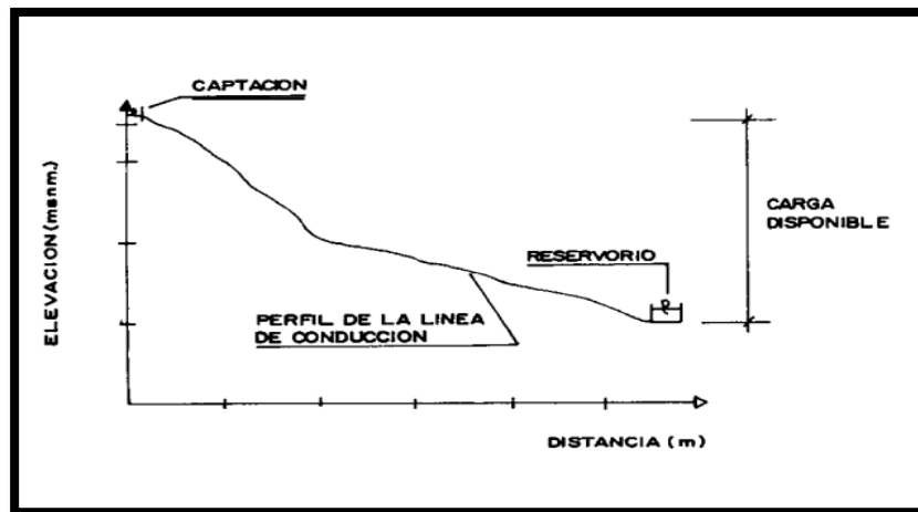
Gráfico 4 Carga disponible en la línea de conducción.
