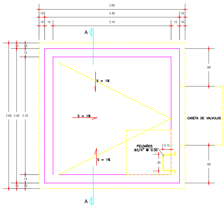
PLANTA ESC: 1/10
