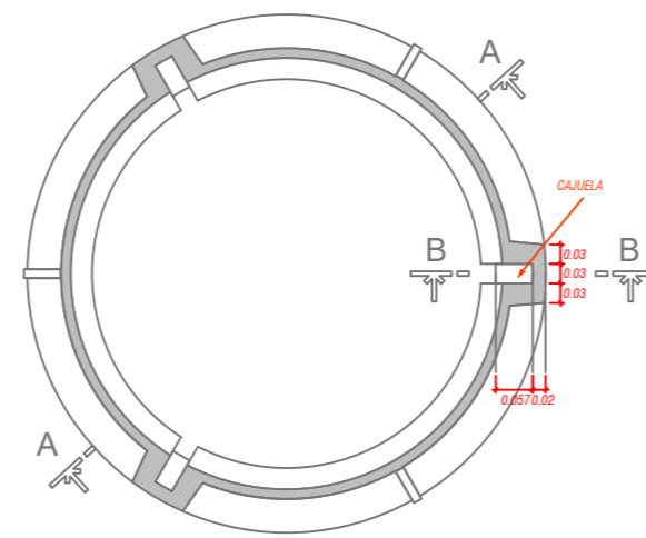
PLANTA: MARCO DE FIERRO FUNDIDO
