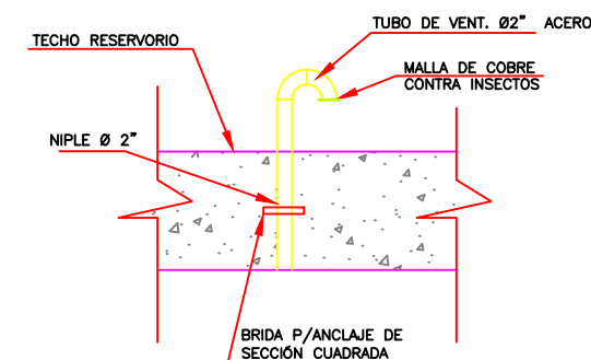
DETALLE DE VENTILACION ESC: 1:15
