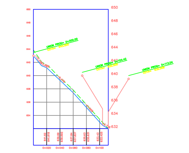
PERFIL DE LA LINEA DE RED DISTRIBUCION SECUNDARIA 1
