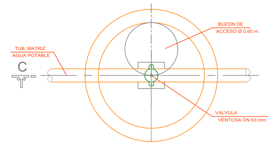
PLANTA Esc: 1/20
