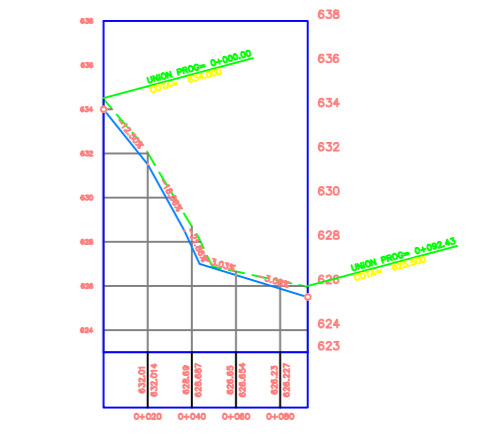
PERFIL DE LA LINEA DE RED DISTRIBUCION SECUNDARIA 4
