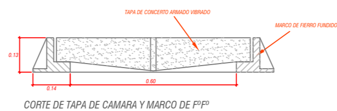
CORTE DE TAPA DE CAMARA Y MARCO DE F° F°
