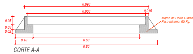
CORTE A-A
