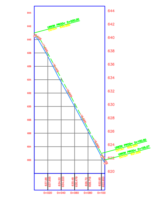
PERFIL DE LA LINEA DE RED DISTRIBUCION SECUNDARIA 5
