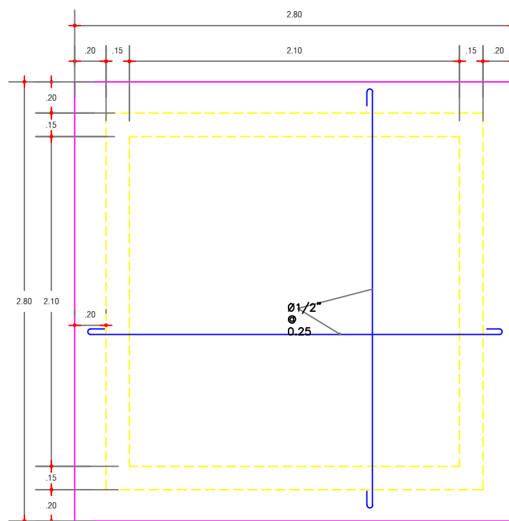
ARMADURA DE FONDO ESC: 1/10
