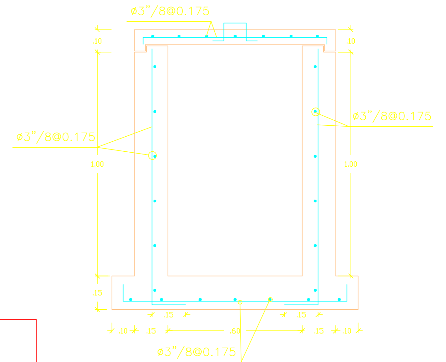
CORTE A-A ESC: 1/10
