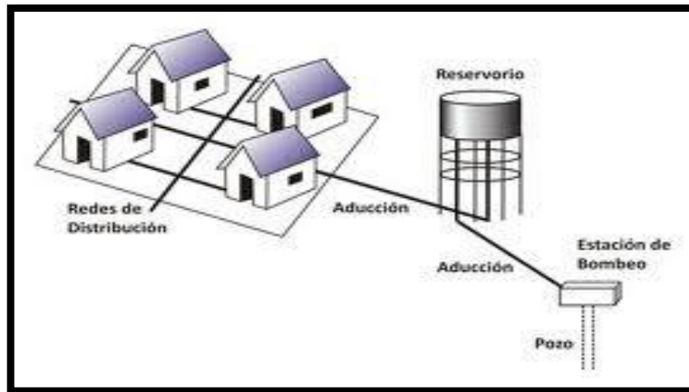
Gráfico 8 Conexiones Domiciliaria
