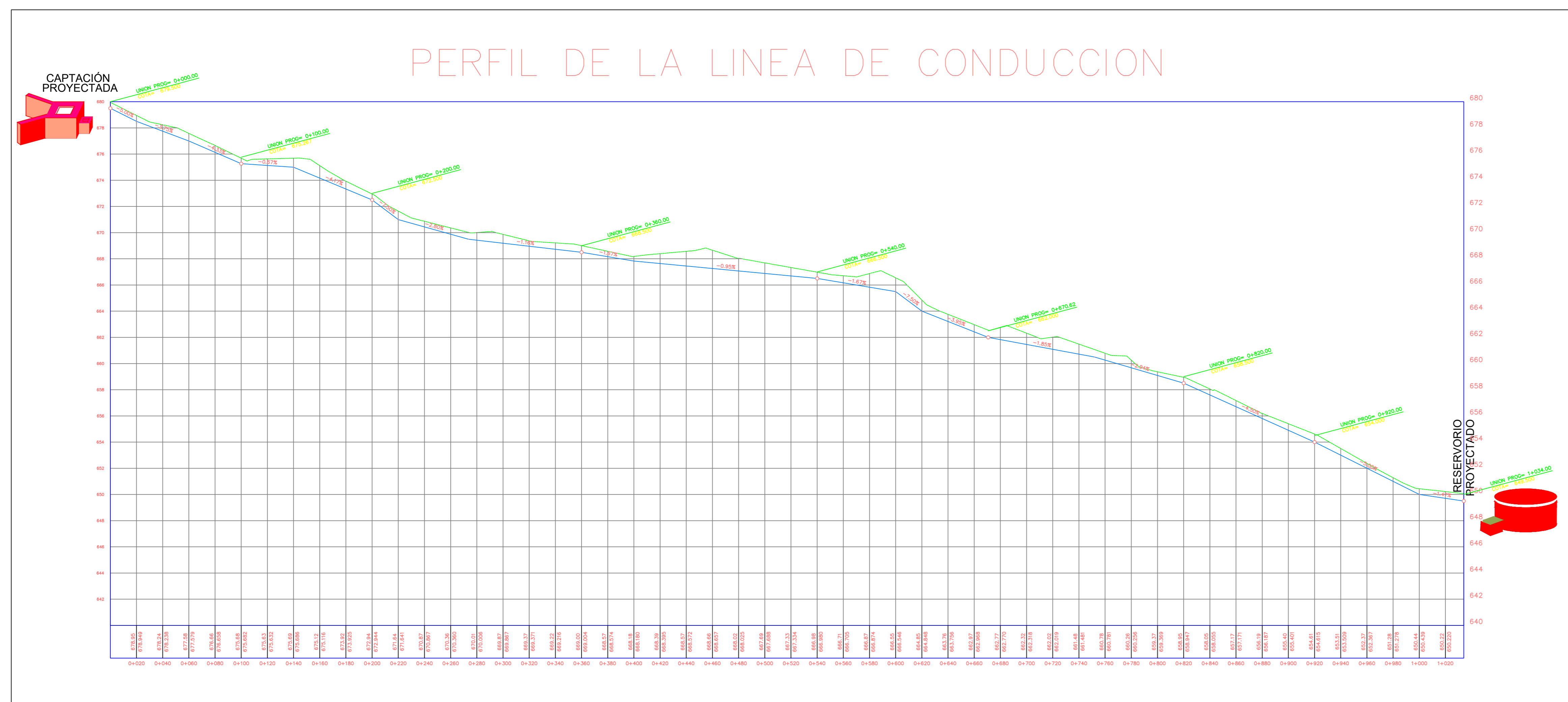
PERFIL LONGITUDINAL - LÍNEA DE CONDUCCIÓN 2020
