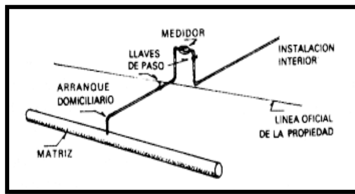
Gráfico 10 Conexiones Domiciliarias
