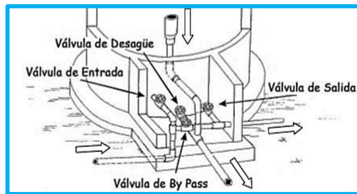
Figura 25. Caseta de válvulas.
