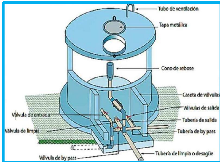
Figura 21. Reservorio de almacenamiento
