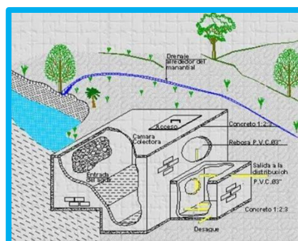
Figura 12. Captación de ladera.
