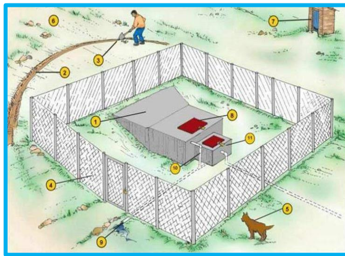
Figura 15. Protección perimetral de captación.
