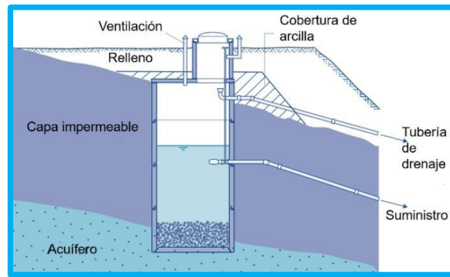
Figura 13. Captación de fondo.
