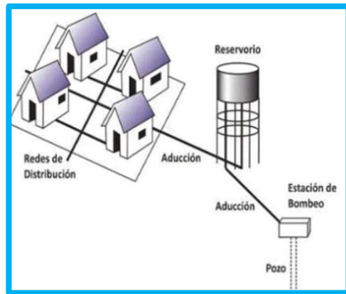
Figura 11. Abastecimiento por bombeo
