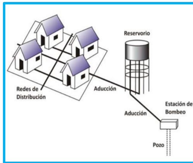
Figura 16. Línea de conducción
