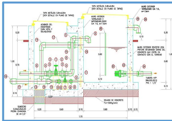
Figura 20. Cámara rompe presión.
