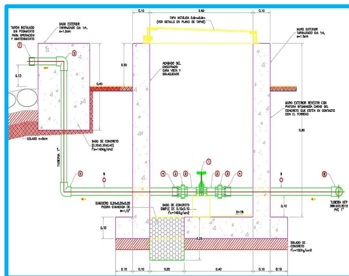
Figura 19. Válvula de purga.
