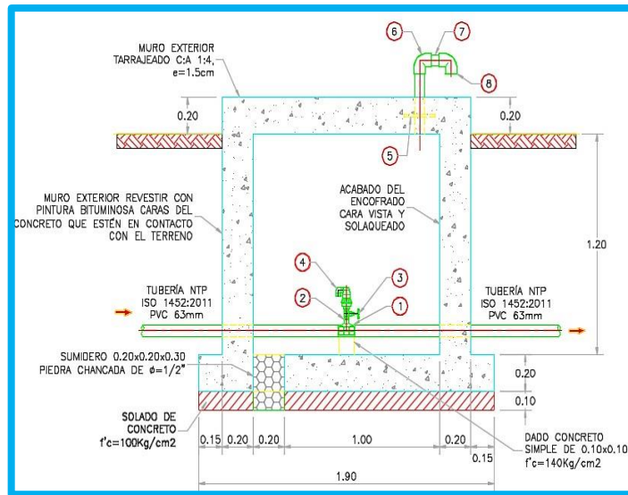
Figura 18. Válvula de aire.
