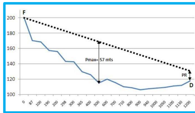
Figura 17. Línea de conducción
