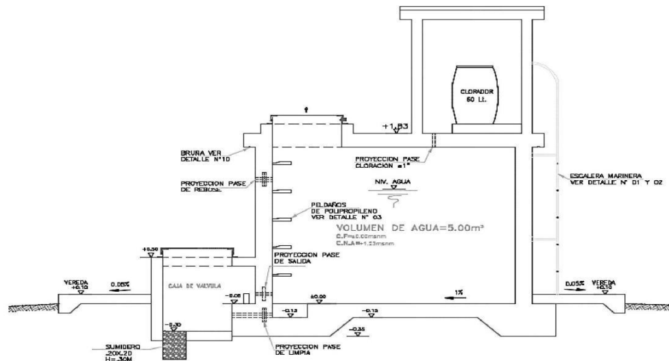
Ilustración N° 03.54. Reservorio de 5 m 3
