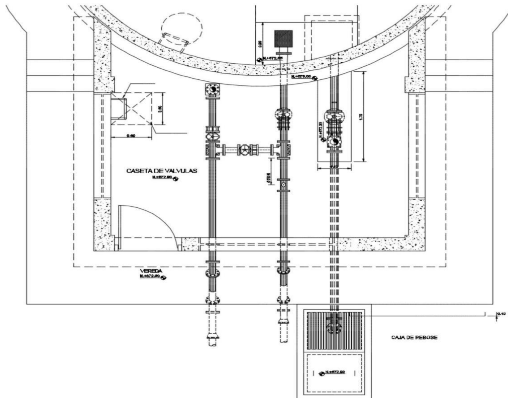
Ilustración N° 03.56. Caseta de válvulas de reservorio de 70 m 3
