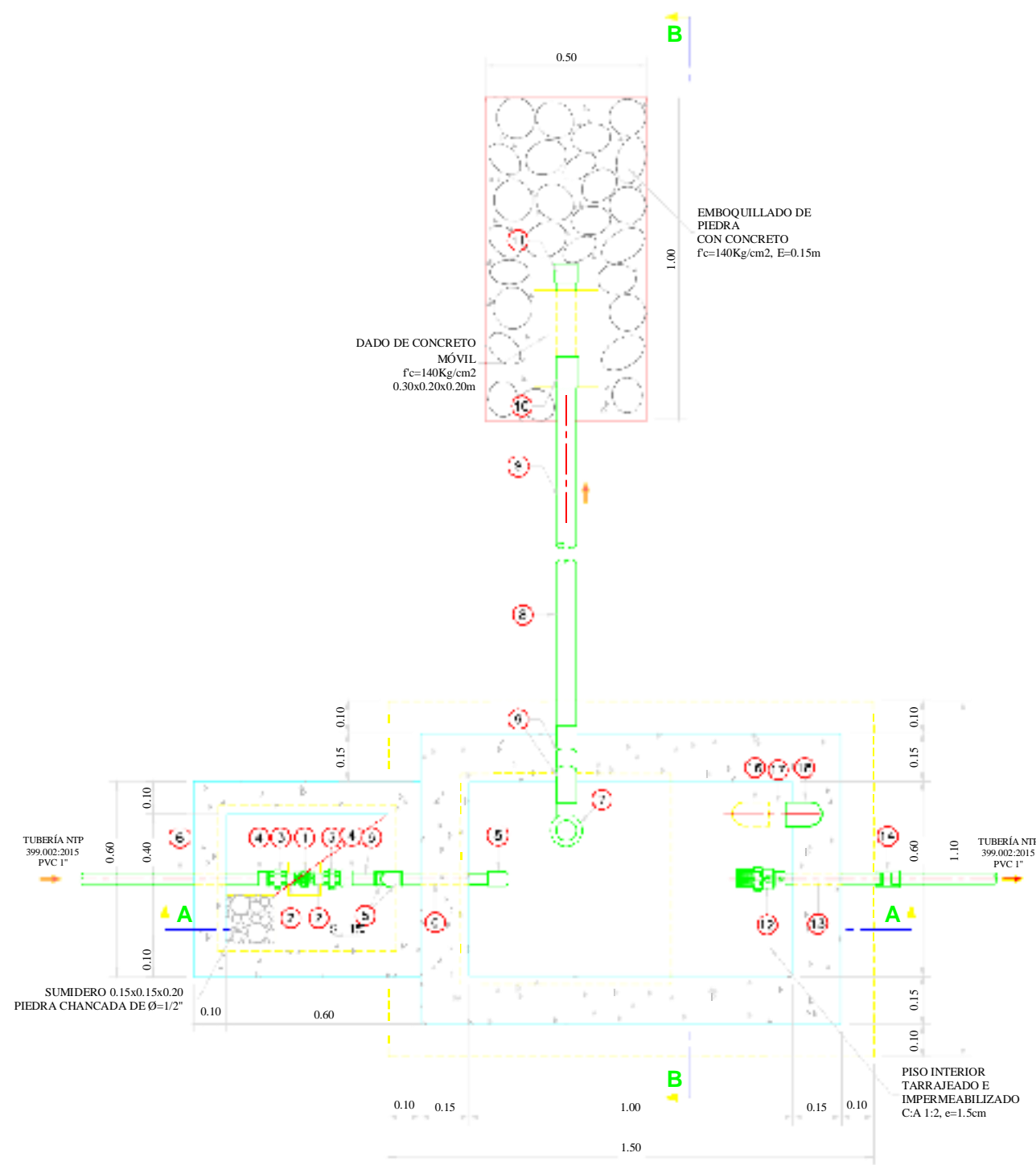
PLANTA 1:12,5
