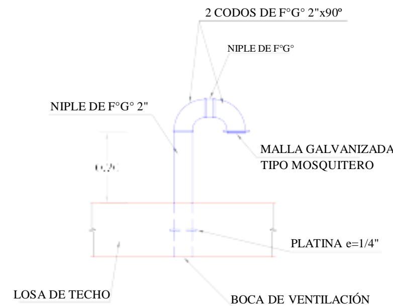
DETALLE DE VENTILACIÓN ESC. 1:10
