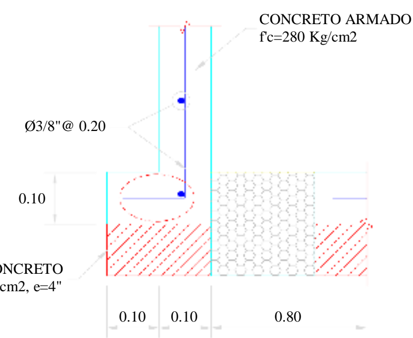
SECCIÓN 1-1 1:5
