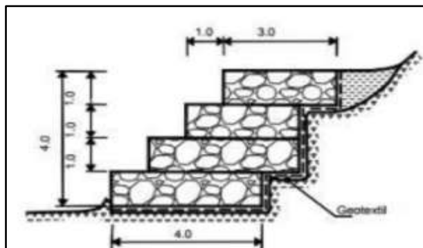
Figura 18: Gaviones
