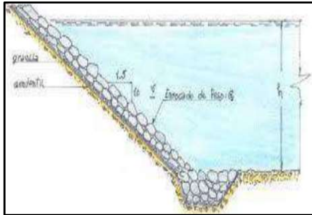
Figura 13: Enrocado.
