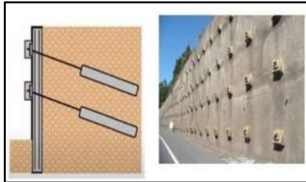
Figura 21: Muro anclado
