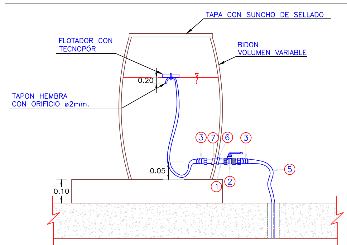
DETALLE DE INSTALACION ESC.:1/10
