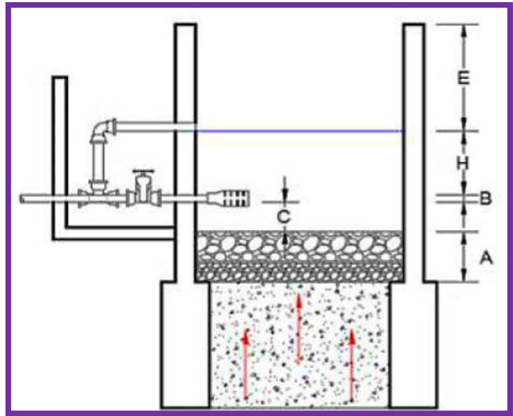
Figura 9. Captación Manantial de fondo
