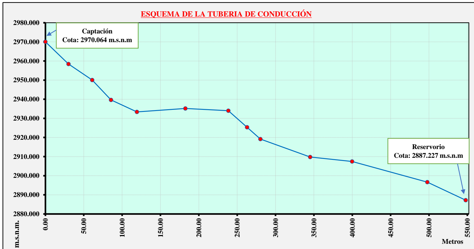
Gráfico 52. Esquema de la tubería de conducción
