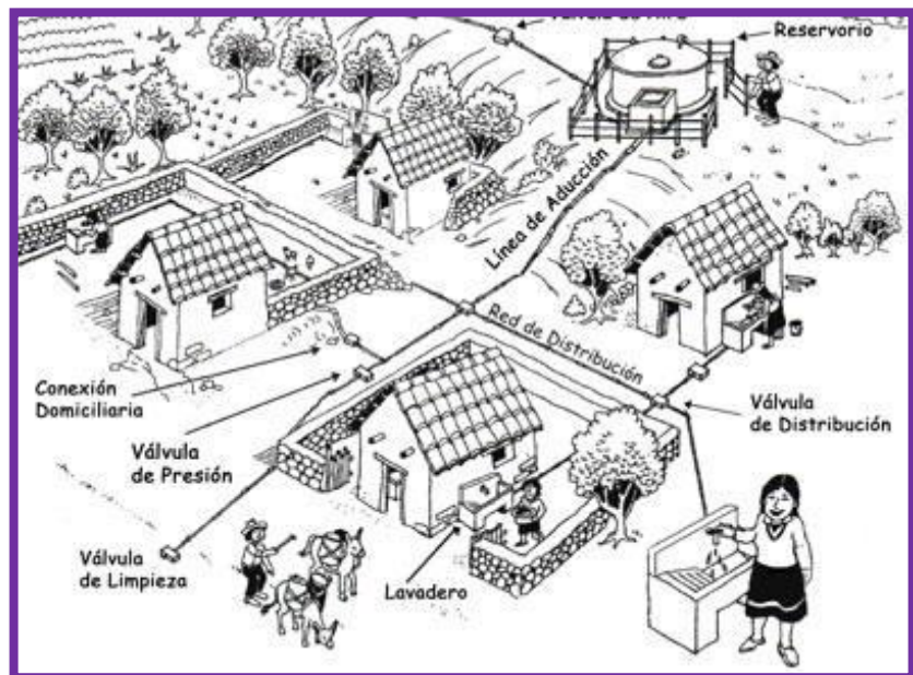
Figura 16. Esquema de una línea de aducción
