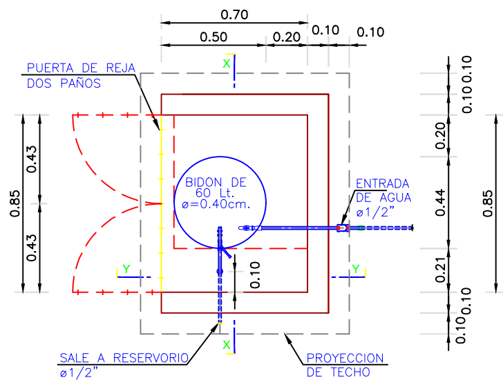
PLANTA ESC. 1:25
