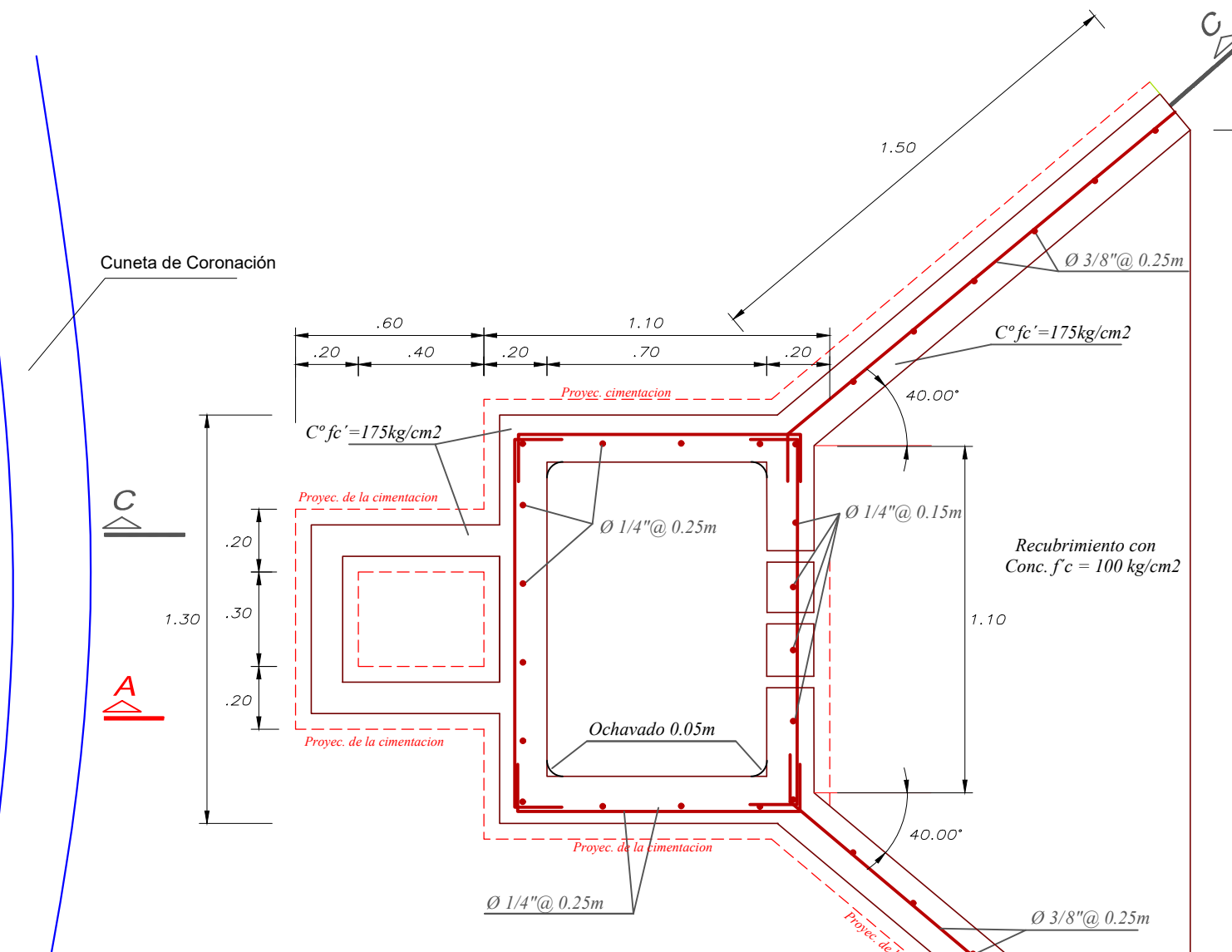
PLANTA (Cimentación-aceros) Esc: 1/20
