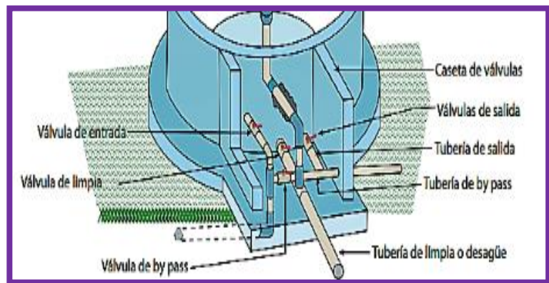
Figura 15. Caseta de válvulas
