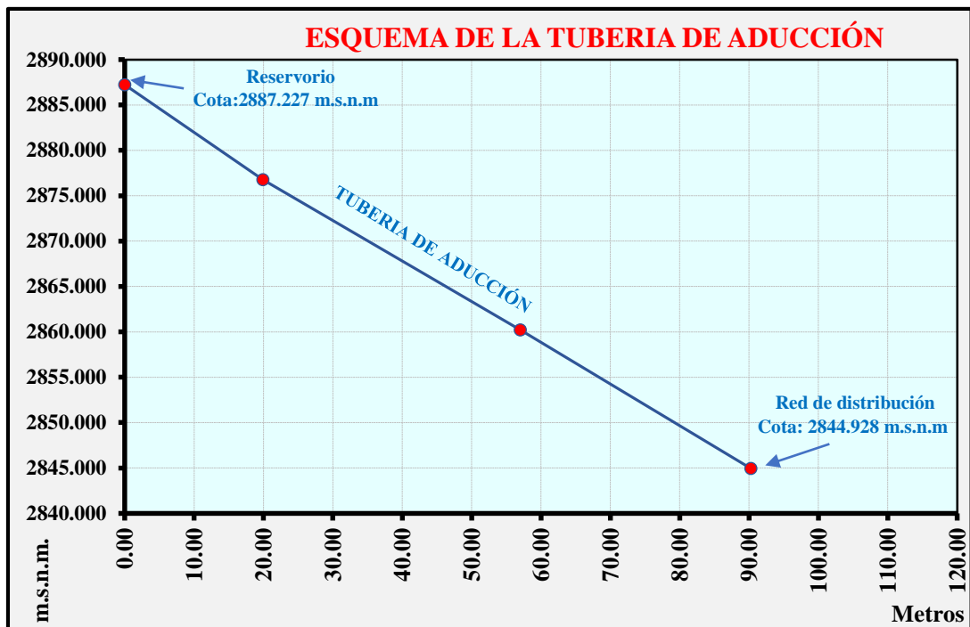
Gráfico 54. Esquema de la tubería de aducción
