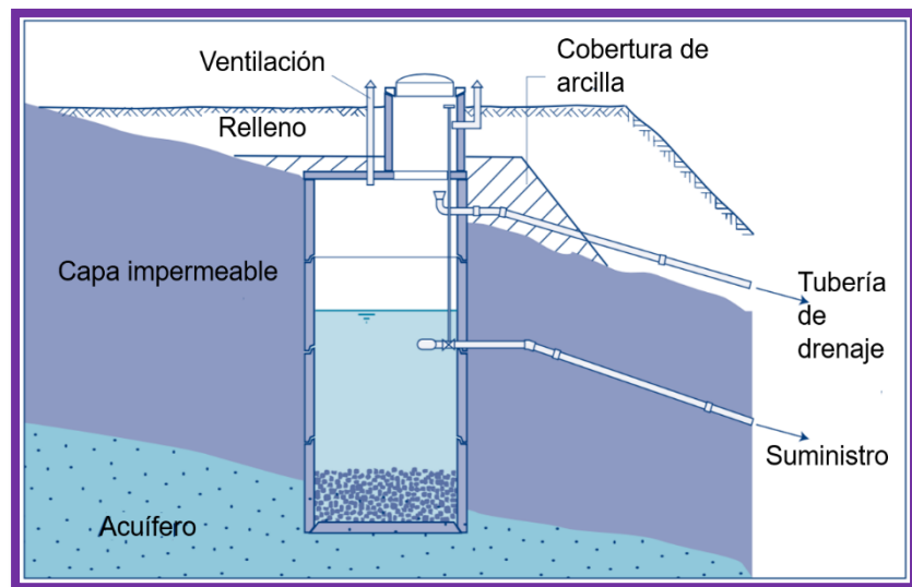
Figura 4. Captación de una fuente subterránea (manantial).
