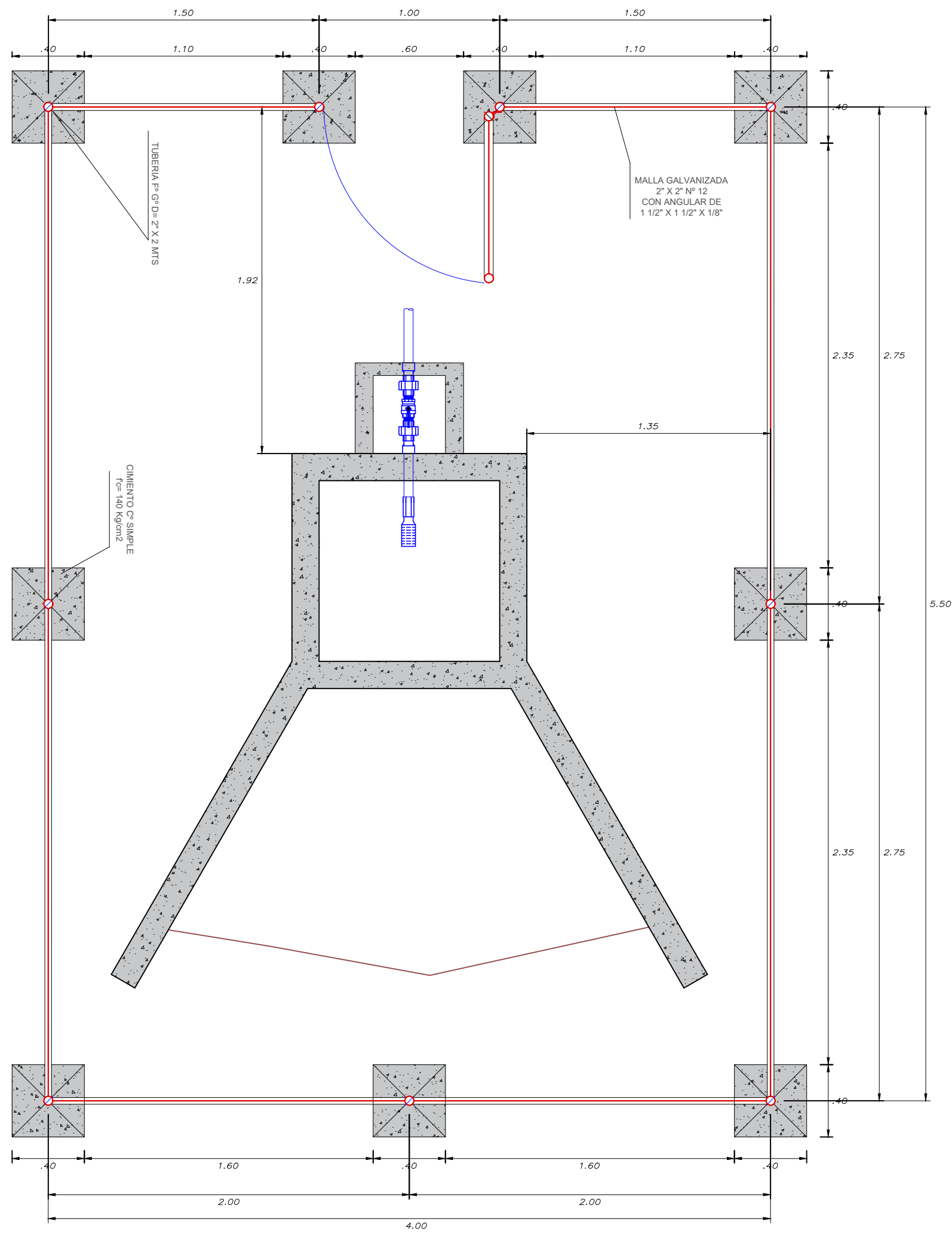
PLANTA CERCO PROTECCION CAPTACION NUEVA ESPERANZA ESC. 1 / 25
