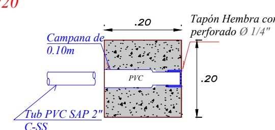
DETALLE A: DADO MOVIL Esc: 1/10
