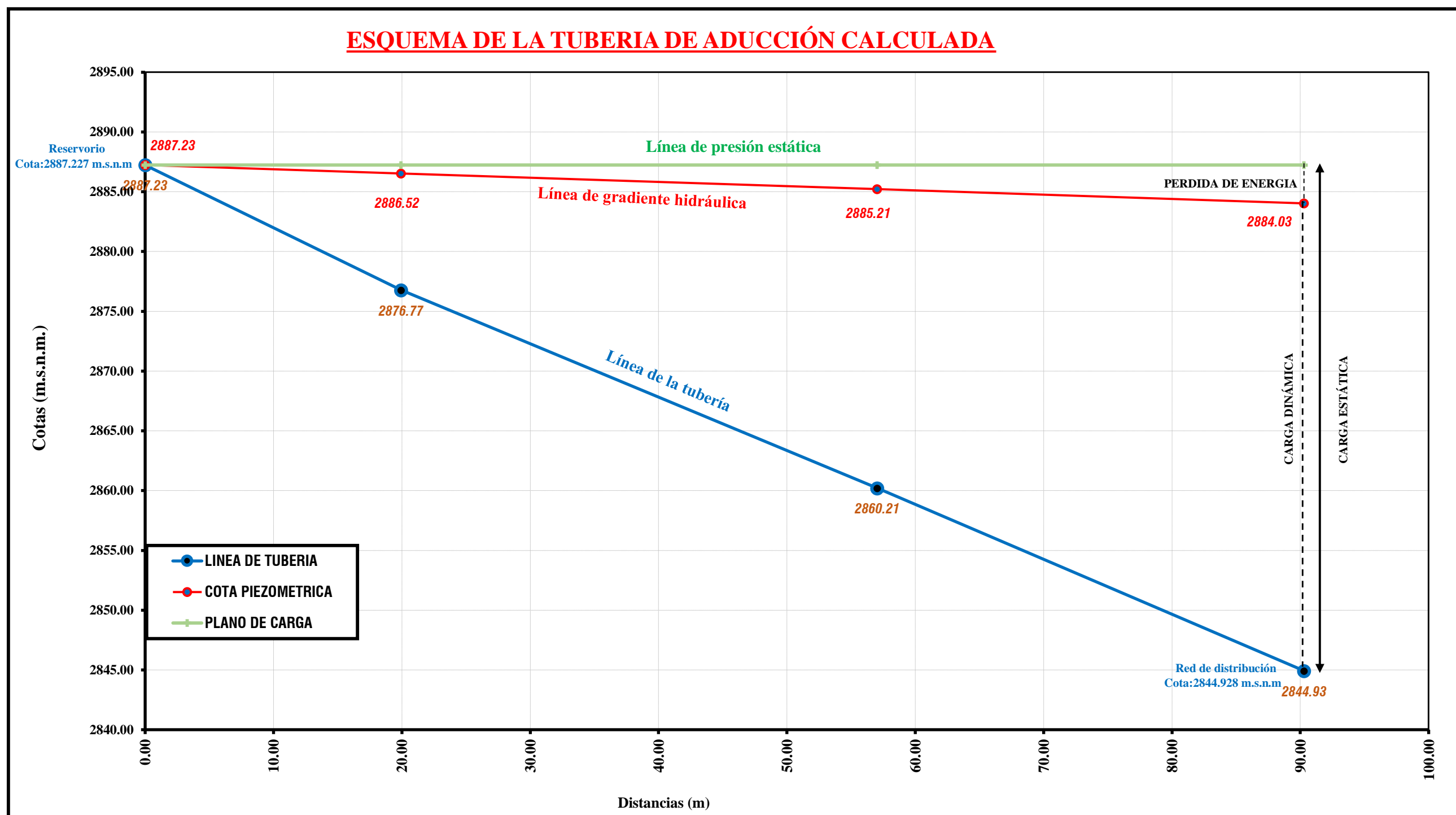
Gráfico 55. Esquema de la tubería de aducción calculada
