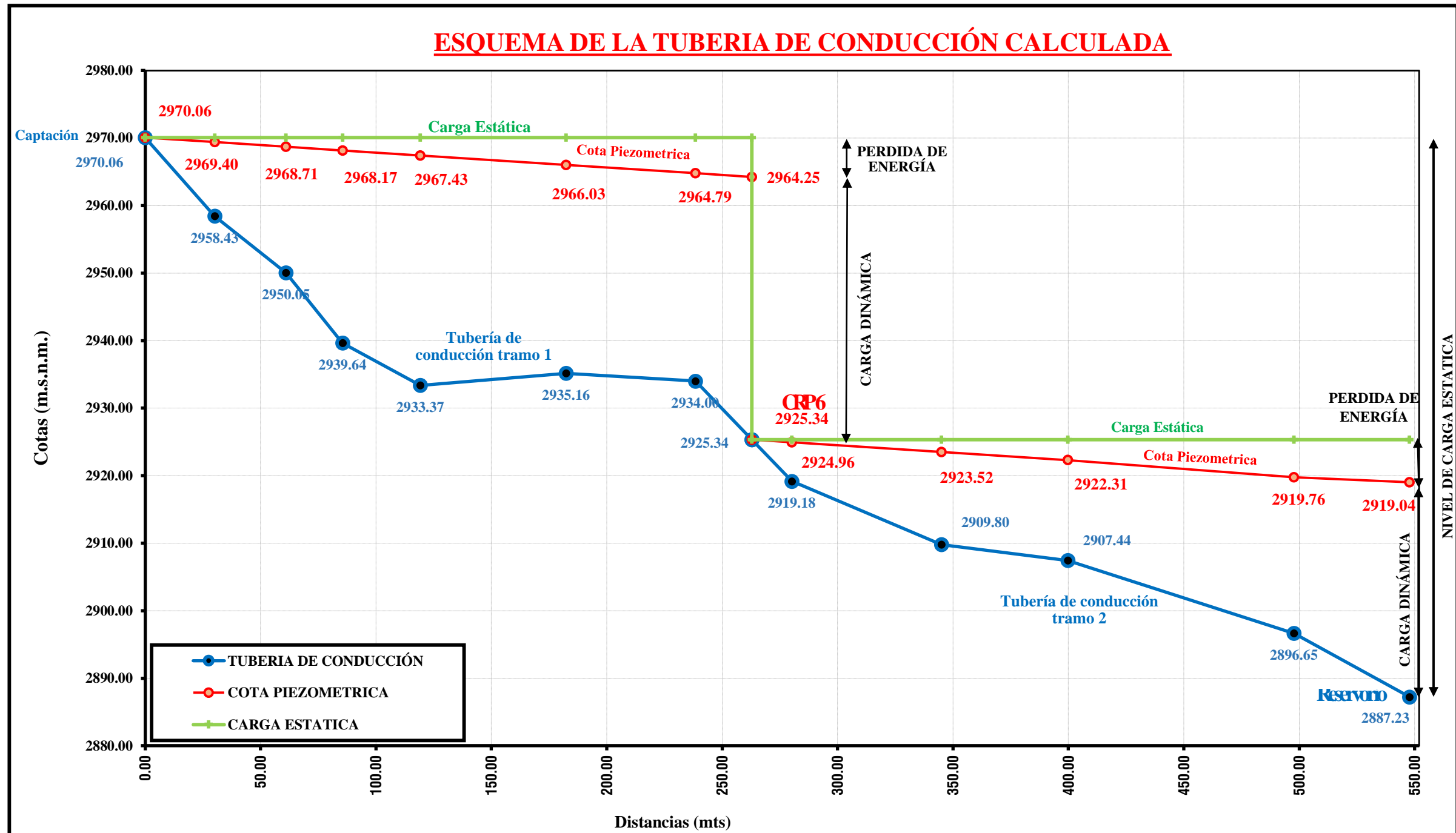
Gráfico 53. Esquema de la tubería de conducción calculada
