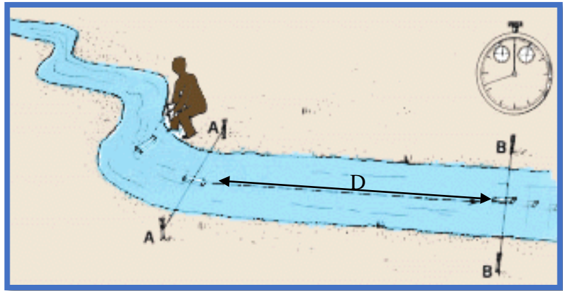
Figura 6. Medición del caudal por el método área - velocidad
