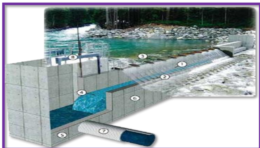
Figura 3. Captación una fuente superficial (río).
