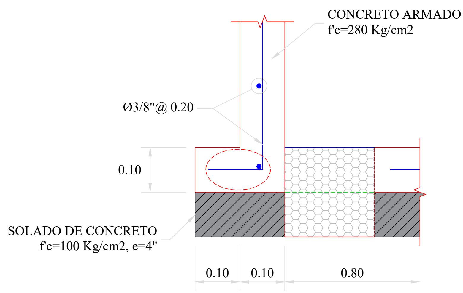
SECCIÓN 1-1 1:5
