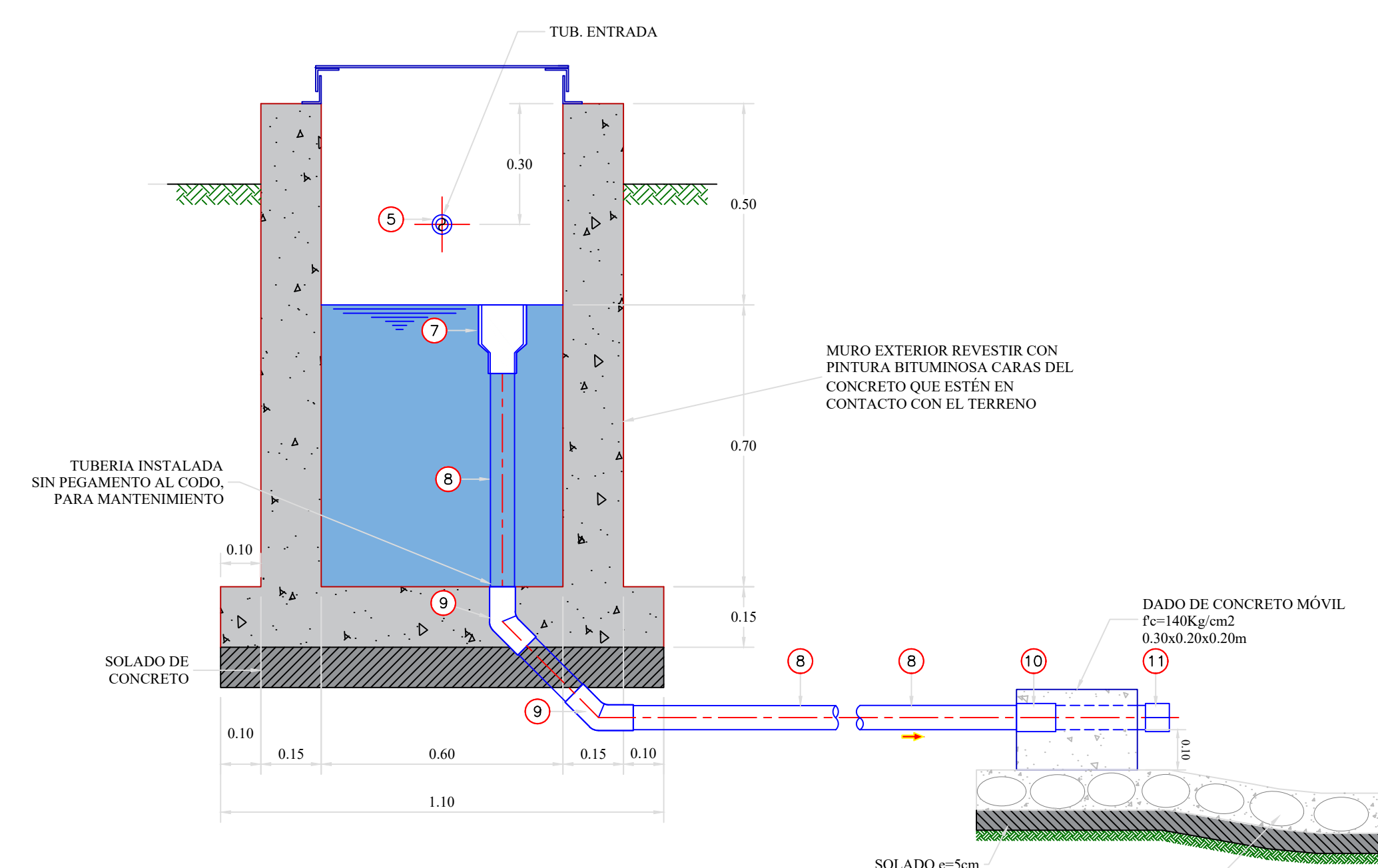
CORTE B-B 1:12,5
