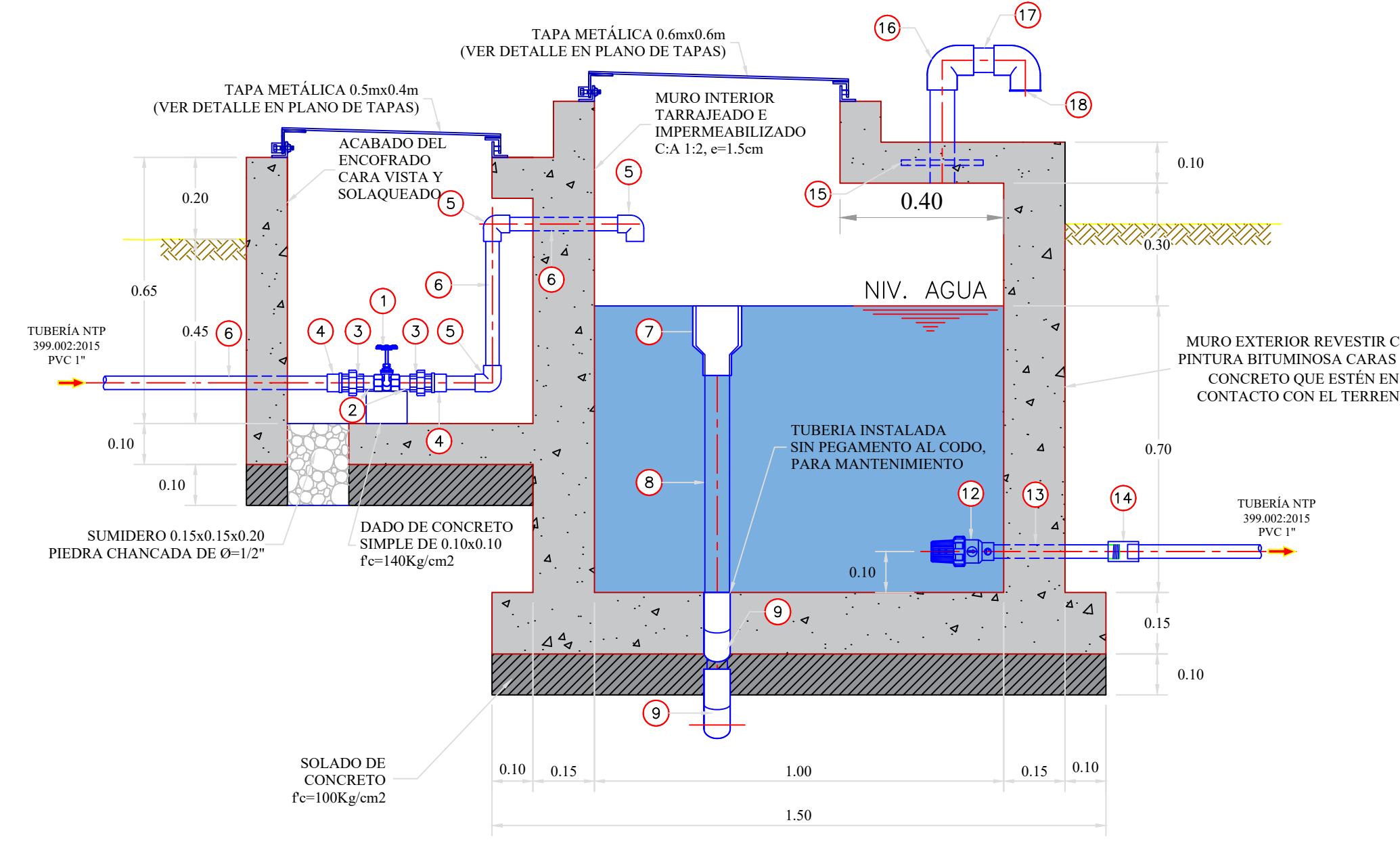
CORTE A-A 1:12,5
