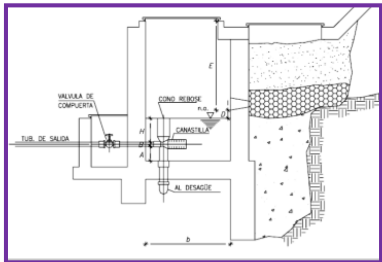
Figura 8. Captación Manantial de Ladera.
