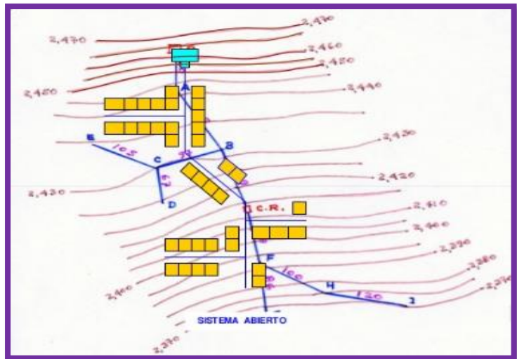
Figura 17. Sistema de una red de distribución abierta
