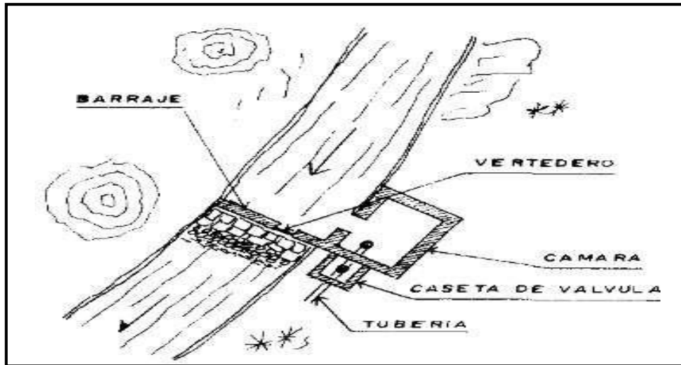
Ilustración 3. Captación de agua superficial.
