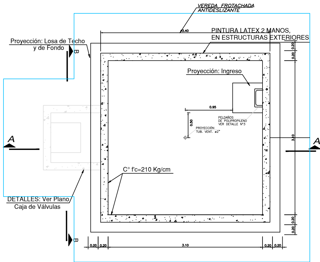
PLANTA ESC. 1:20
