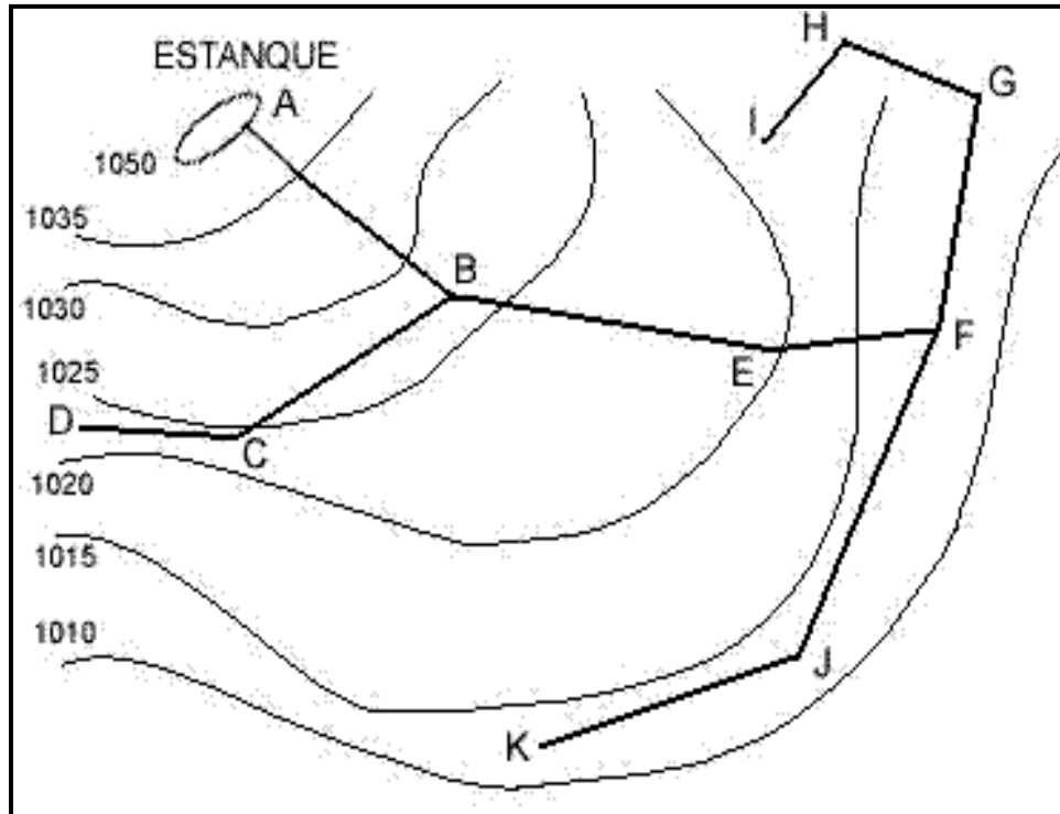
Ilustración 17. Red de Distribución de Agua-Sistema ramificado.
