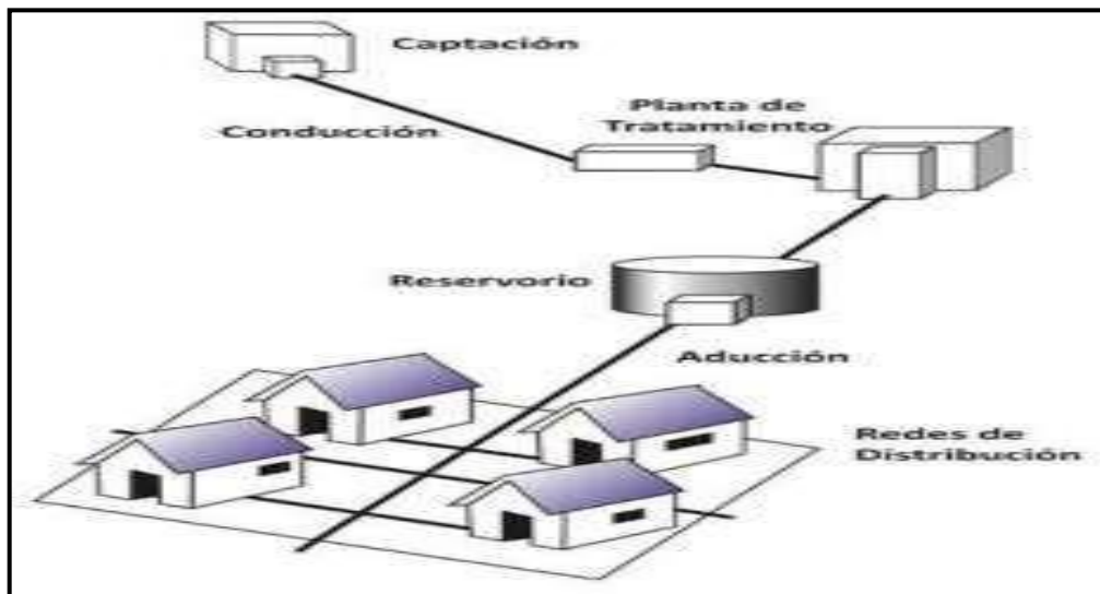
Ilustración 5. Sistema por gravedad con tratamiento.
