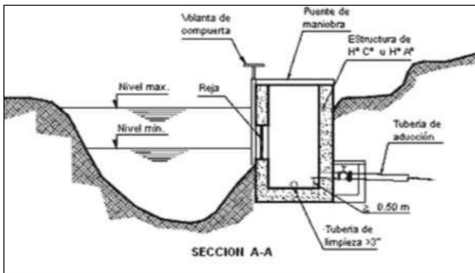
Ilustración 8. Vista de perfil de una toma lateral.
