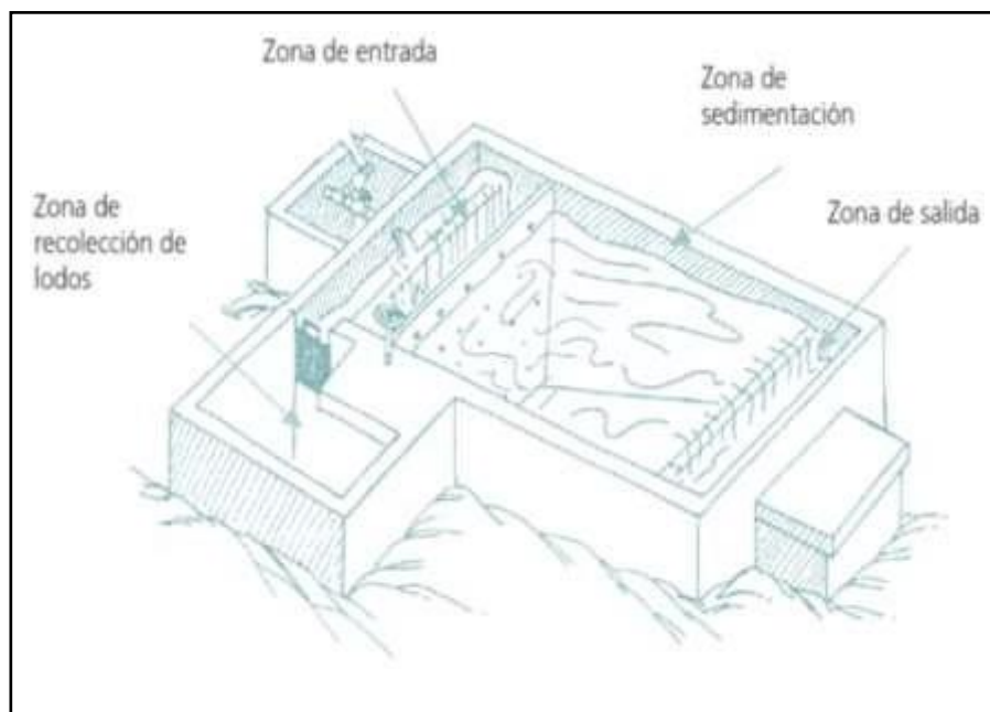
Ilustración 13. Vista de planta, de una Planta de Tratamiento de Agua. Fuente: Diapositivas de Partes y funciones del sistema de agua potable. Programa buena gobernanza (22) .
