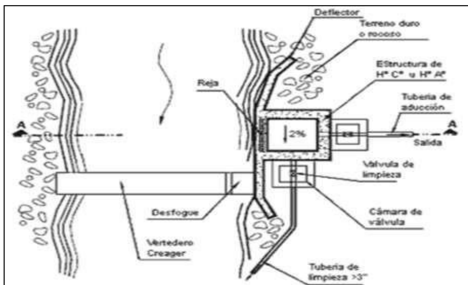
Ilustración 7. Vista de planta de una toma lateral.
