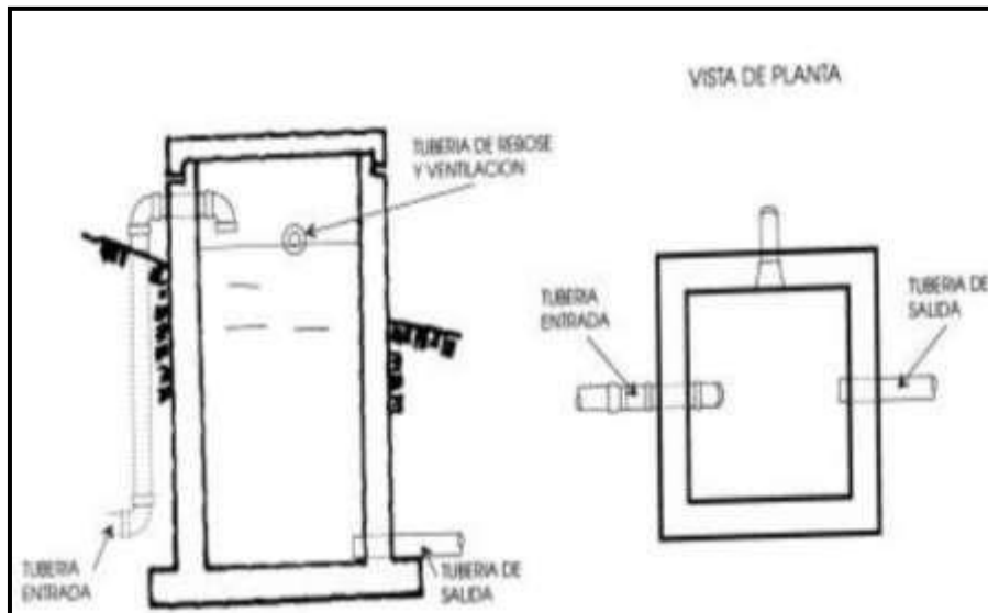
Ilustración 9. Cámara Rompe presión.
