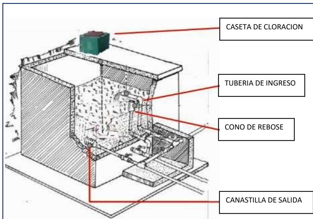
Ilustración 15. Partes Internas del Reservorio.
