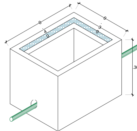
ISOMETRICO DE CAJA DE CONCRETO DE 0.30m x 0.40m PREFABRICADA
