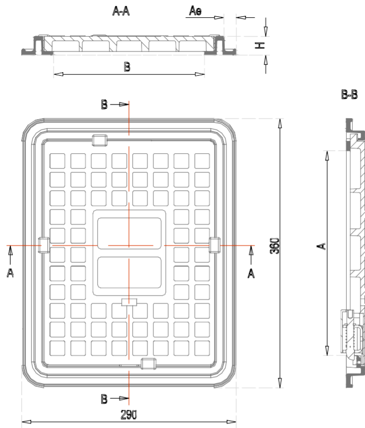
TAPA TERMOPLASTICA
