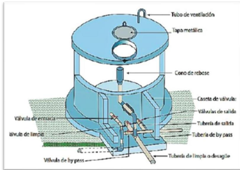
Grafico 7. Esquema y partes de un reservorio.
